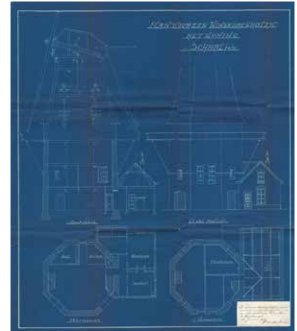
Bouwtekening van de molen, 1910
